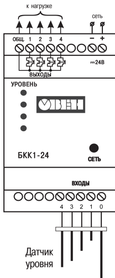
Рисунок 5.3 – Схема подключения БКК1-24 Рисунок 5.4 – Схема подключения БКК1-220
