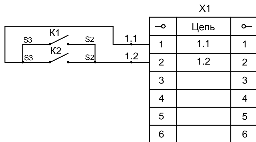
Схема электрическая соединений
